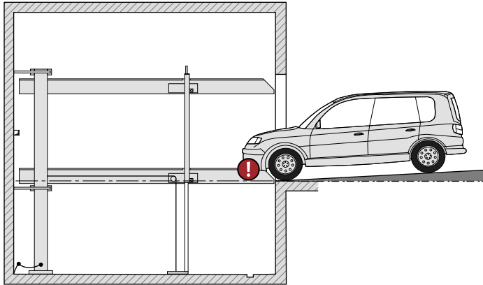
max. 3% spadek
