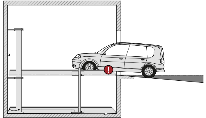
max. 10% wznios
