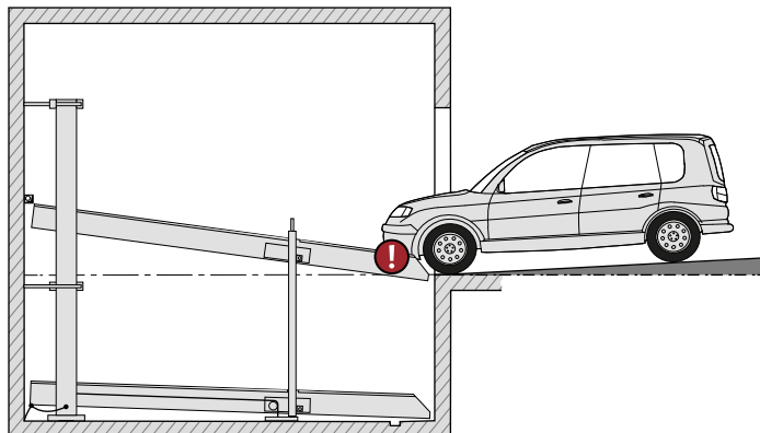
max. 10% spadek
