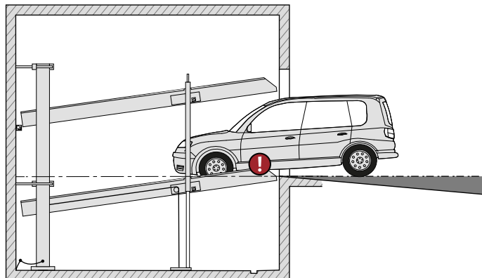
max. 2% wznios
